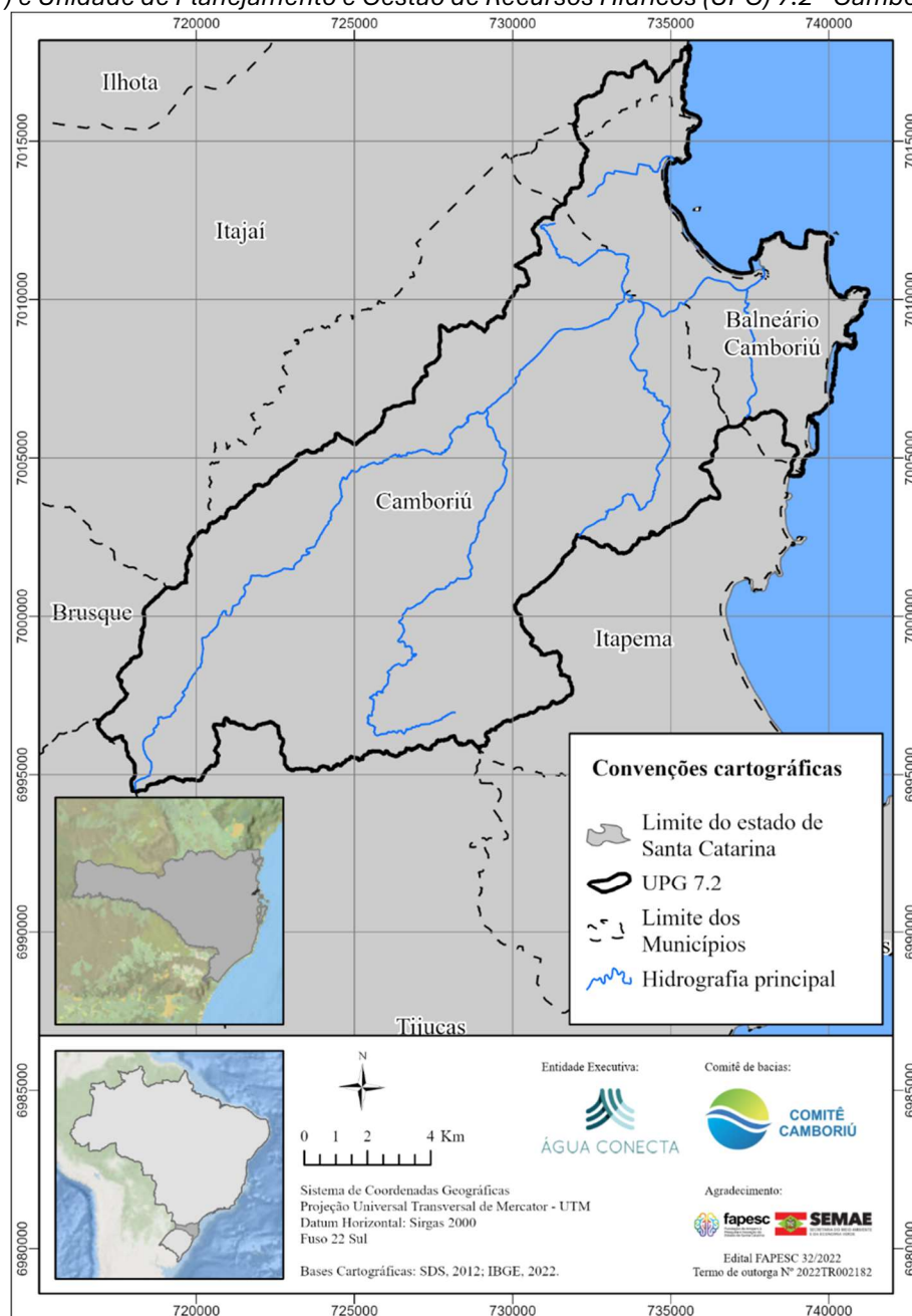
Figura 1: Localização da área de abrangência do Comitê Camboriú, na Região Hidrográfica do Vale do Itajaí (RH 07) e Unidade de Planejamento e Gestão de Recursos Hídricos (UPG) 7.2 - Camboriú.
